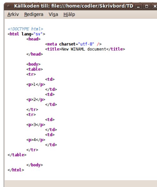
Figur 2. Den genererade HTML-koden.
