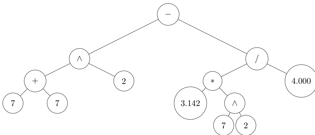
Figure 1: Ett uttrycksträd
