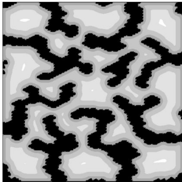
Flood fill
