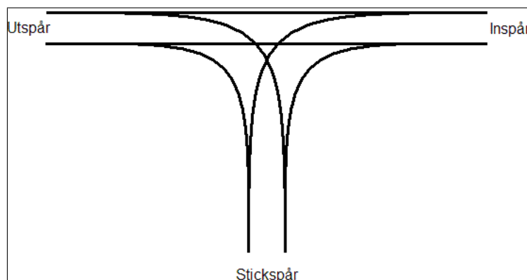
Figur 1: Järnvägsalgoritmen med in-, ut- och stickspar.
